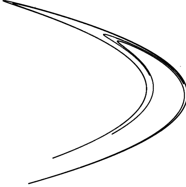
FIGURE 1 – Attracteur de l'application de Hénon. Pour des paramètres bien choisis, l'ensemble représenté est compact invariant et possède la propriété suivante : pour tout point x au voisinage, d(f^n(x), \cdot) \xrightarrow[n \rightarrow +\infty]{} 0 .
